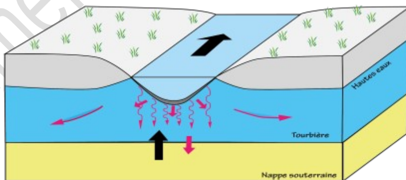
Schéma des relations entre rivière, nappe souterraine et nappe de la tourbe
