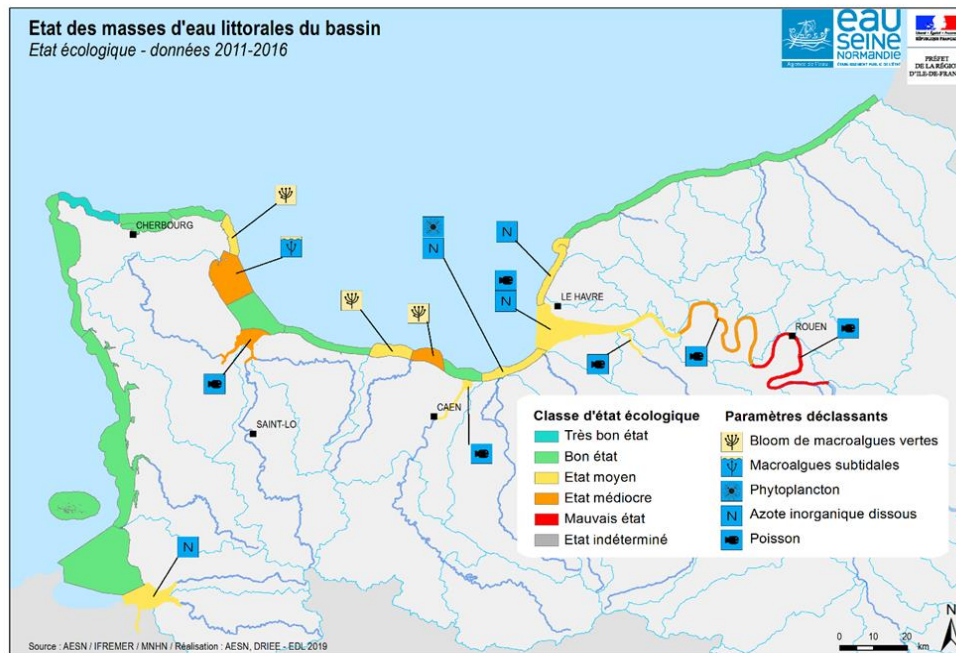
Carte 34 : Etat des masses d'eau littorales
