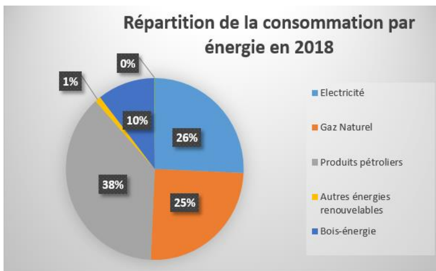
Figure 7 : Consommation d'énergie en 2018 - Répartition par énergie, Source : Observatoire Régionale Énergie-Climat-Air de Normandie
