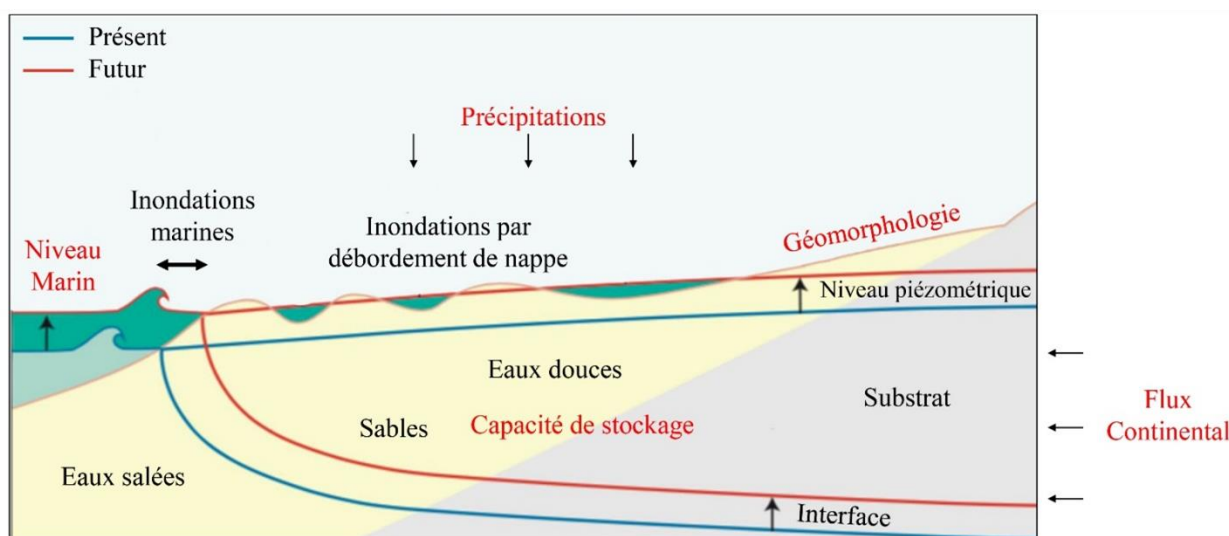
Figure 3 : Remontée du biseau salé liée au changement climatique (A Gauvain, Université de Rennes)
