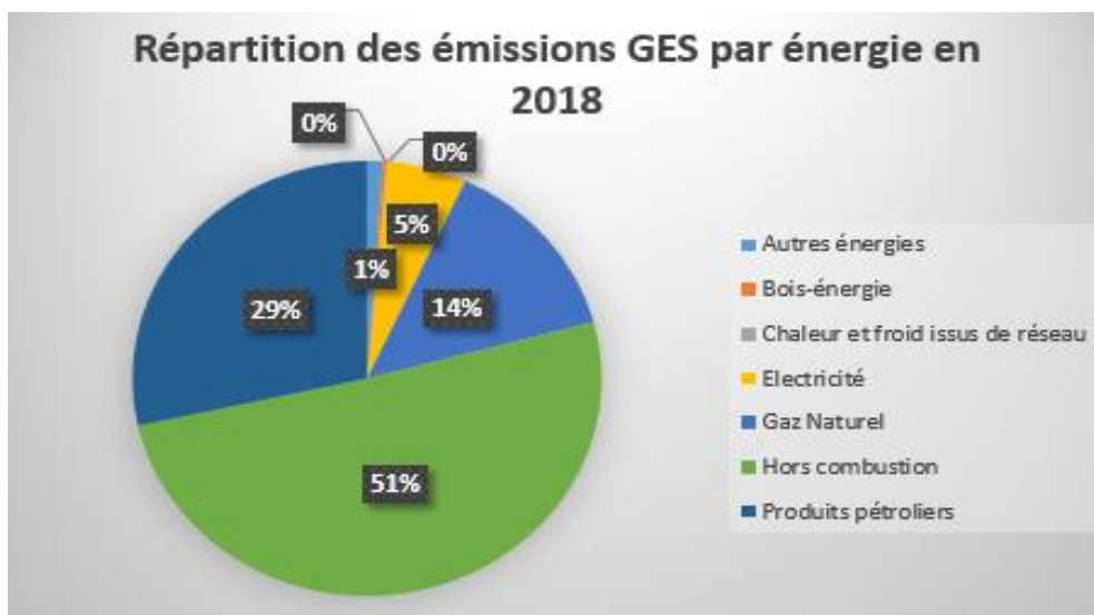
Figure 5 : Émissions de gaz à effet de serre en 2018 - Répartition par énergie, Source : Observatoire Régionale Énergie-Climat-Air de Normandie
