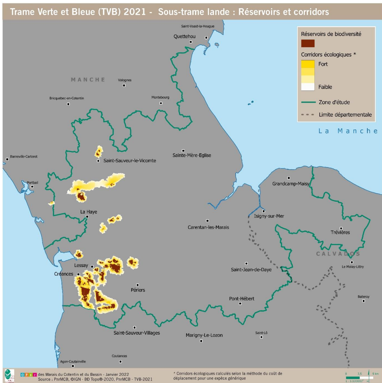
Carte 27 : Réservoirs et corridors de la sous-trame lande
